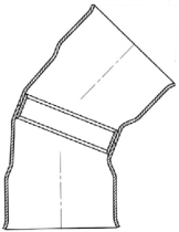
45° Bend HxH
